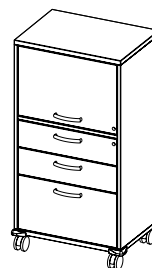
Hauteur 1 148 (3 HC), largeur 600, profondeur 436 mm
