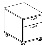
9 UH Avec plumier intégré, hauteur 542, largeur 430, profondeur 600/800 mm
